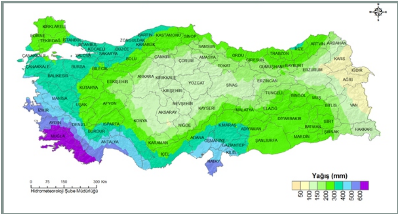
Şekil-4 Türkiye Kış Mevsimi Alansal Yağış Haritası
