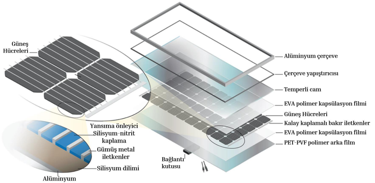
 ekil 2: k-Si FV G ne  Panelinin Yapısı
